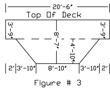
End view exc. dim. for 17 x 37 Em.
